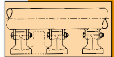
Breite Schlegel
